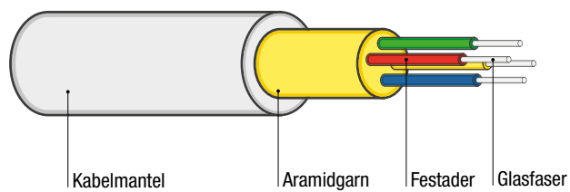
Aufbau FTTH-Kabel 2.8mm
