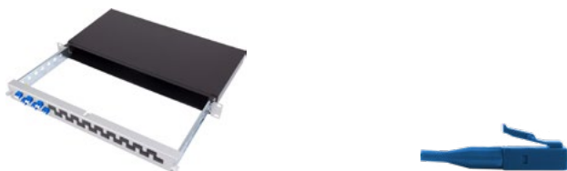
Tête de câbles 19" pour câbles préconfectionnés Patch-KEV LC/PC
