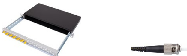
Tête de câbles 19" pour câbles préconfectionnés Patch-KEV ST/PC
