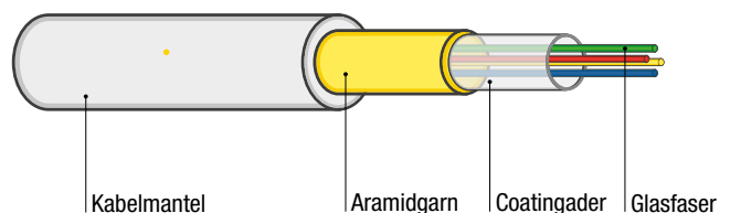
Aufbau FTTH-Kabel 2.2mm
