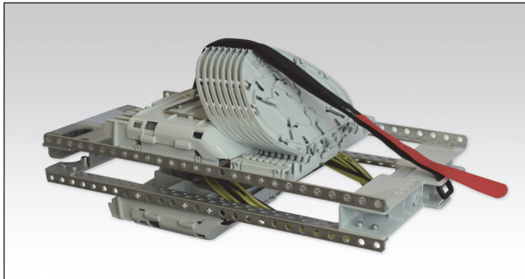
1 Kassettenrahmen mit SC Kassetten für 48 Glasfasern
